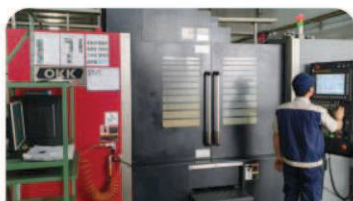
立形マシニングセンター モデル: OKK VM760R
